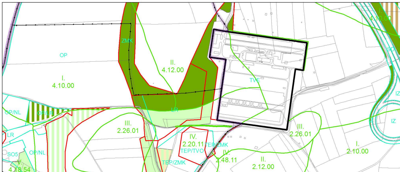
Výkres č. 20 – Vyhodnocení záborů ZPF a PUPFL (LPF), platný stav k 1. 1. 2017
